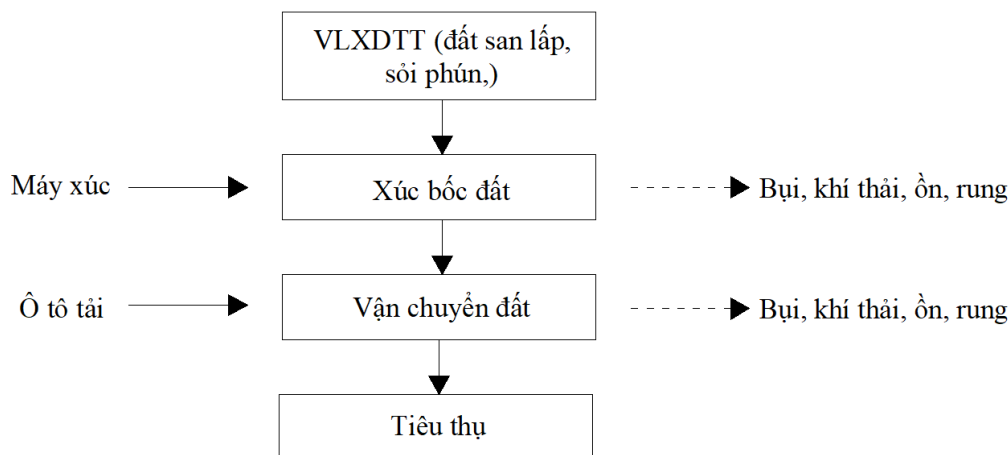
Hình 1.2. Sơ đồ công nghệ khai thác của dự án
